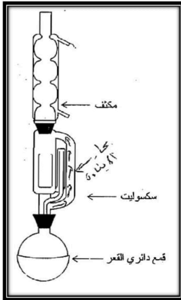
(جهاز السكسوليت)
